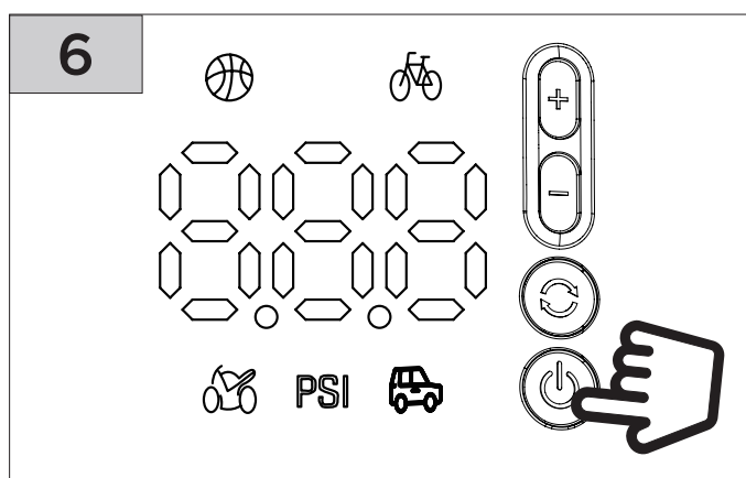
6. Appuyez une fois sur le bouton Marche/Arrêt pour procéder au gonflage. La pompe s'arrête automatiquement une fois la pression définie atteinte
